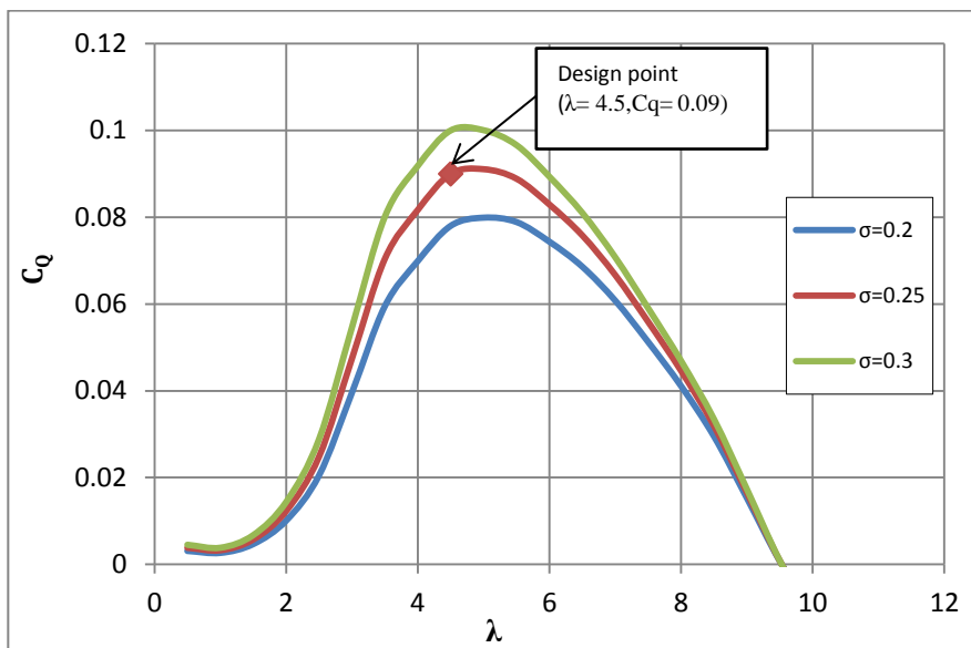
الشكل (9) العلاقة بين معامل عزم الدوران ( C_Q ) ونسبة السرعة الطرفية ( \lambda ) ( 0.2 \leq \sigma \leq 0.3 , C_{d0}=0.017 )
