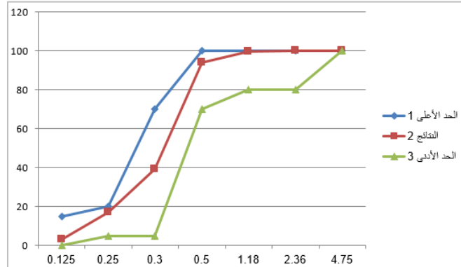
شكل 1: منحنى التحليل المنخلي للركام الناعم
