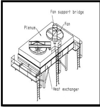
شكل (2) أبراج السحب الإجباري
