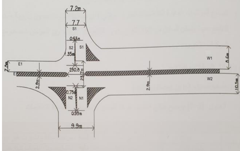
شكل (1) عرض الحارات والارصفة علي التقاطع
