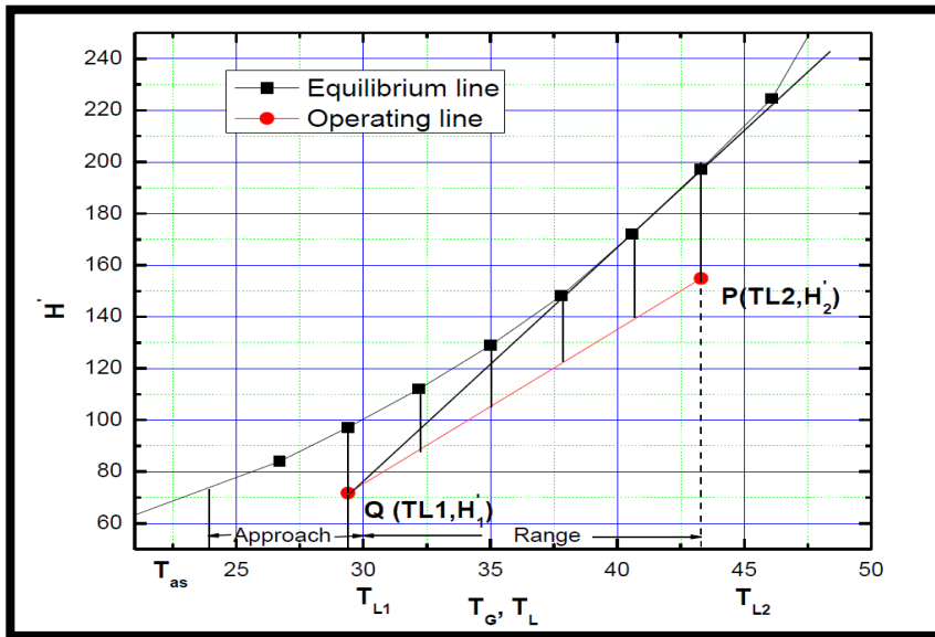
شكل (6) خط التشغيل و منحني الاتزان
