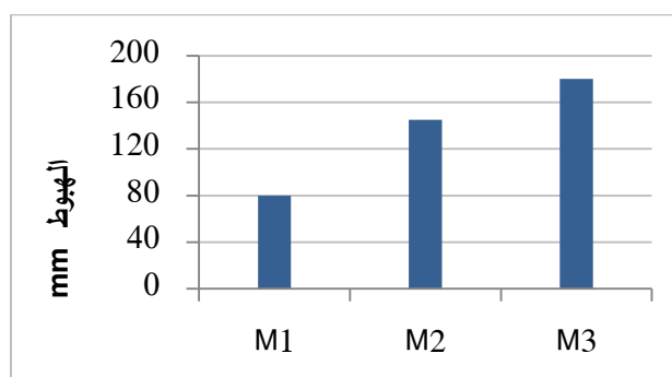
شكل 3: مقدار الهبوط لجميع أنواع العينات
