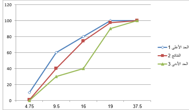
شكل 2: منحني التحليل المنخلي للركام الخشن الخليط
